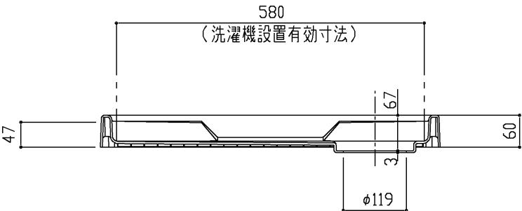
断面A-A
